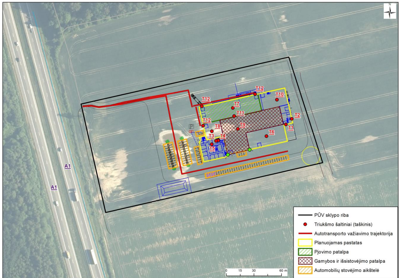
5.3.1 pav. Triukšmo šaltinių išdėstymas.
