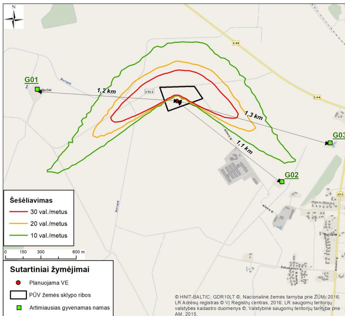
5.5.1 pav. Planuojamos VE sukiamo šešėliavimo izolinių grafinis atvaizdavimas.
