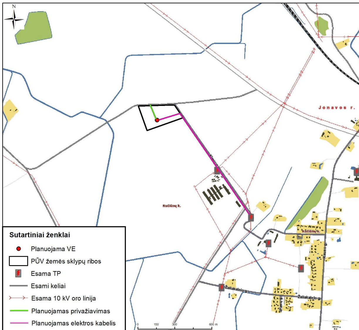
4.3.1. pav. Esamos ir preliminarai planuojamos inžinerinės infrastruktūros schema.
