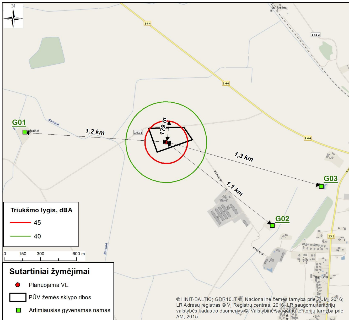
5.3.1 pav. Prognozuojamo PŪV triukšmo lygio izolinijos.
